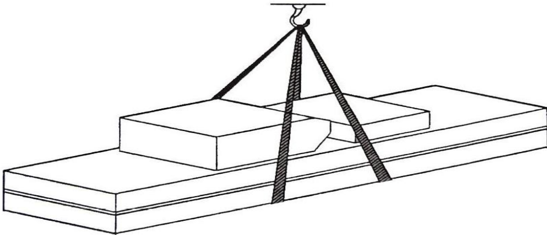
Рис. 1 Строповка оборудования
